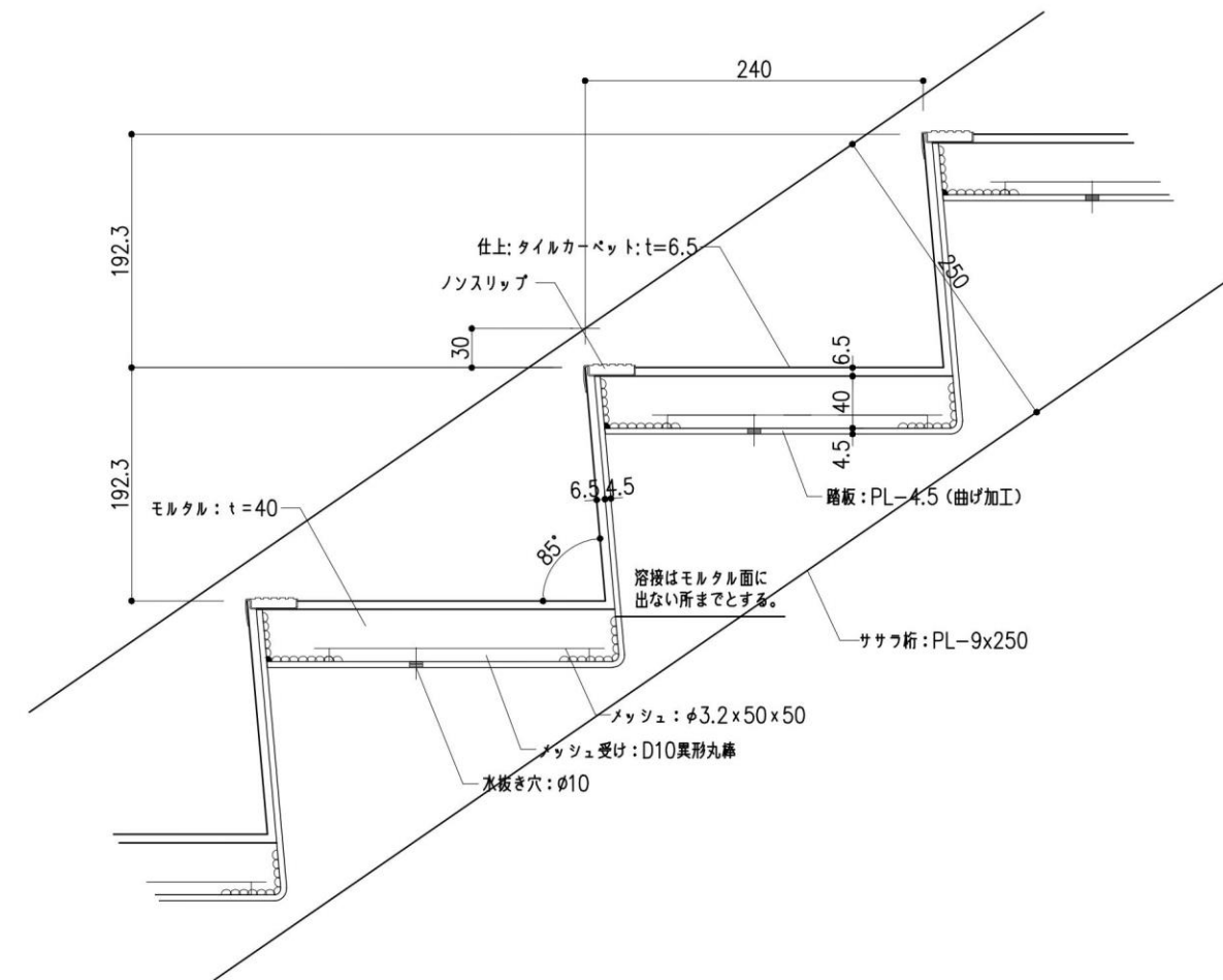
段部詳細図
