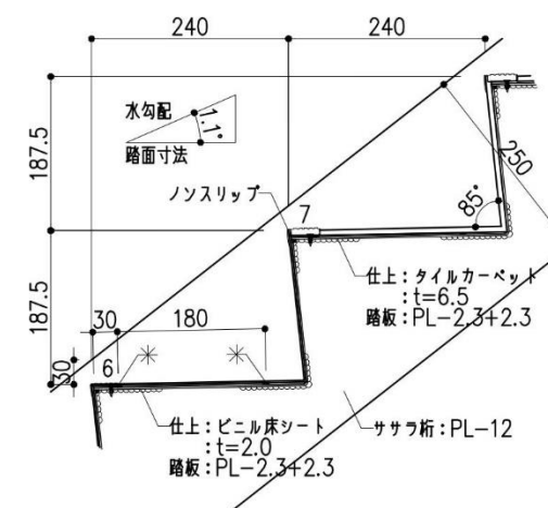
SS 階段 段部詳細図
