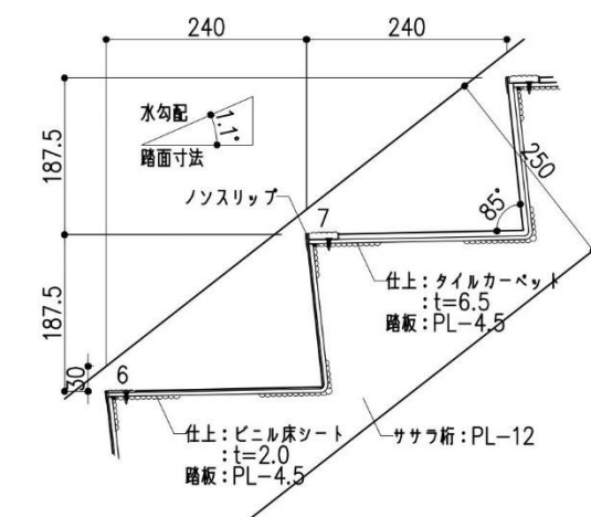
直貼り階段 段部詳細図
